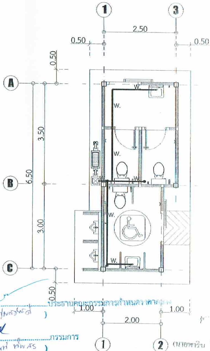
แปลนห้องน้ำทิ้ง
