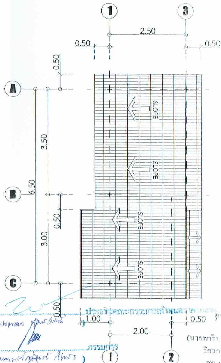
แปลนหลังคา
