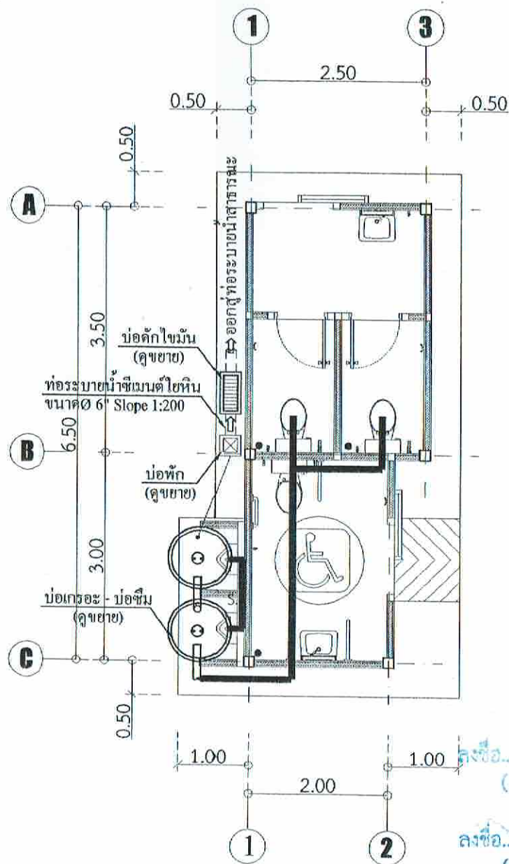
แปลนห้องน้ำเสีย
