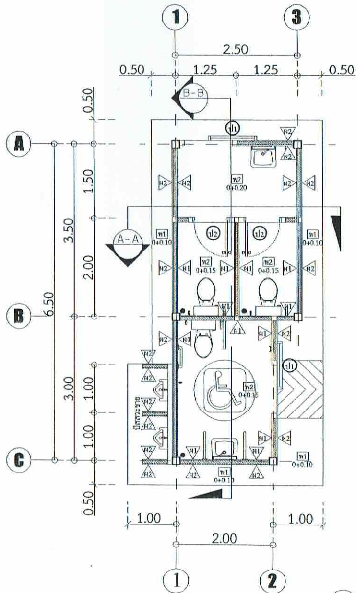
แปลนพื้น
